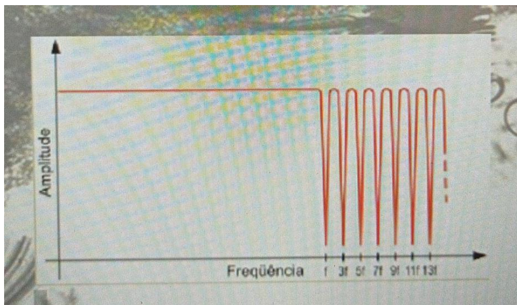
Resposta do filtro pente
