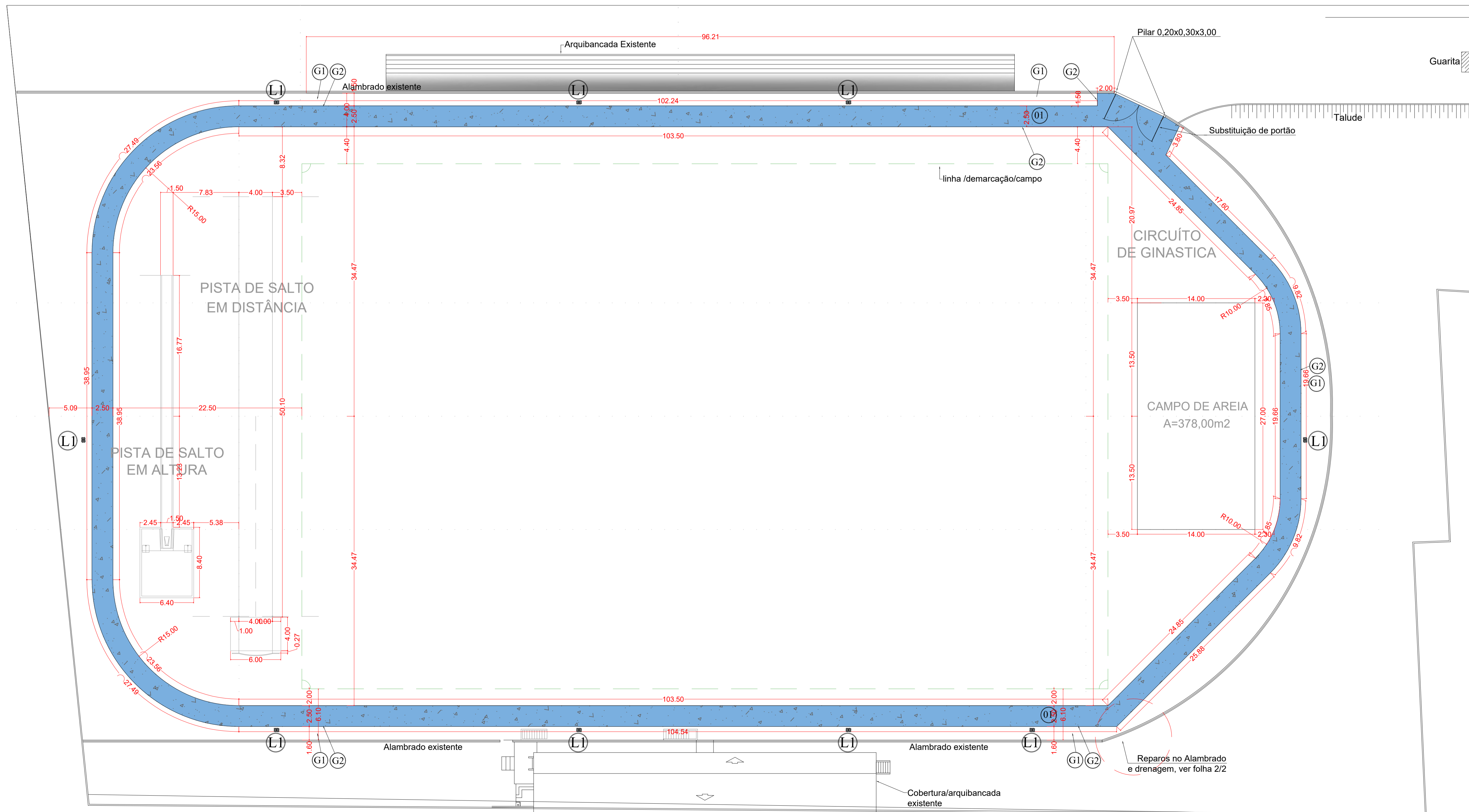
PLANTA/IMPLANTAÇÃO ESC. 1:250
