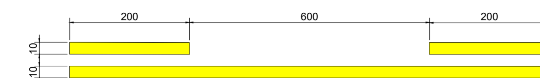
MODELO I FAIXA DUPLA TRACEJADA E CONTÍNUA
