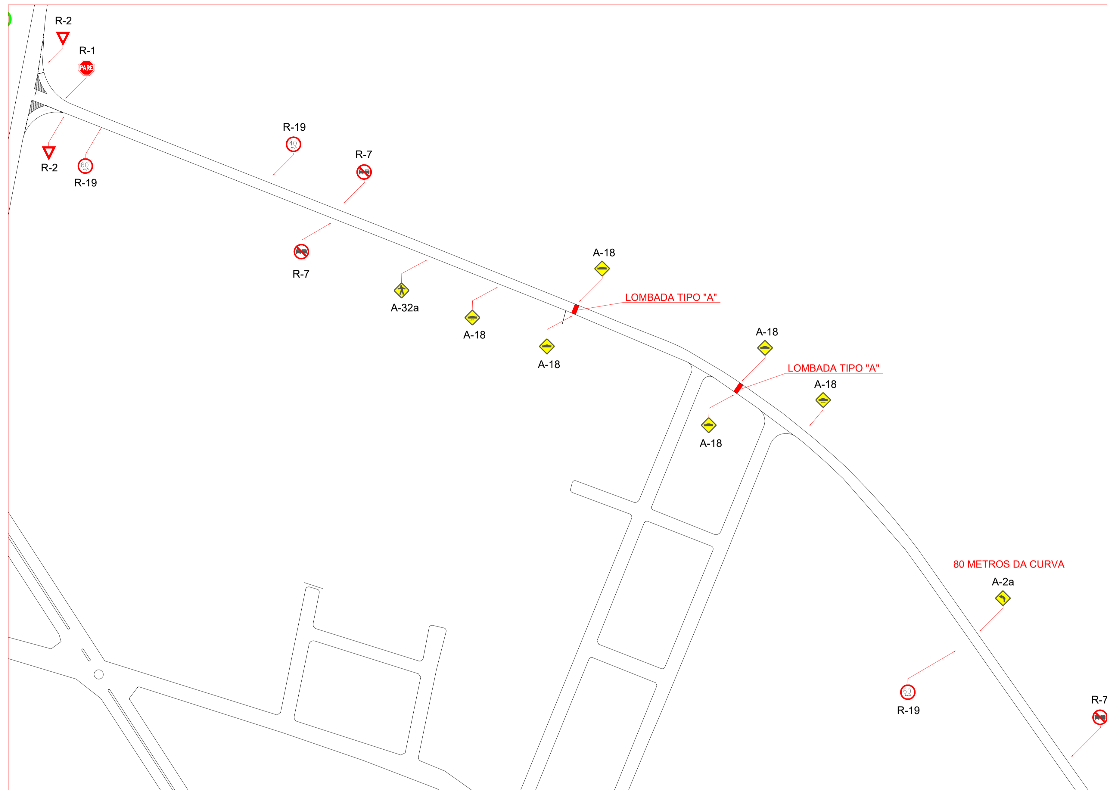
DEMARCAÇÃO - SPA - 498/284
