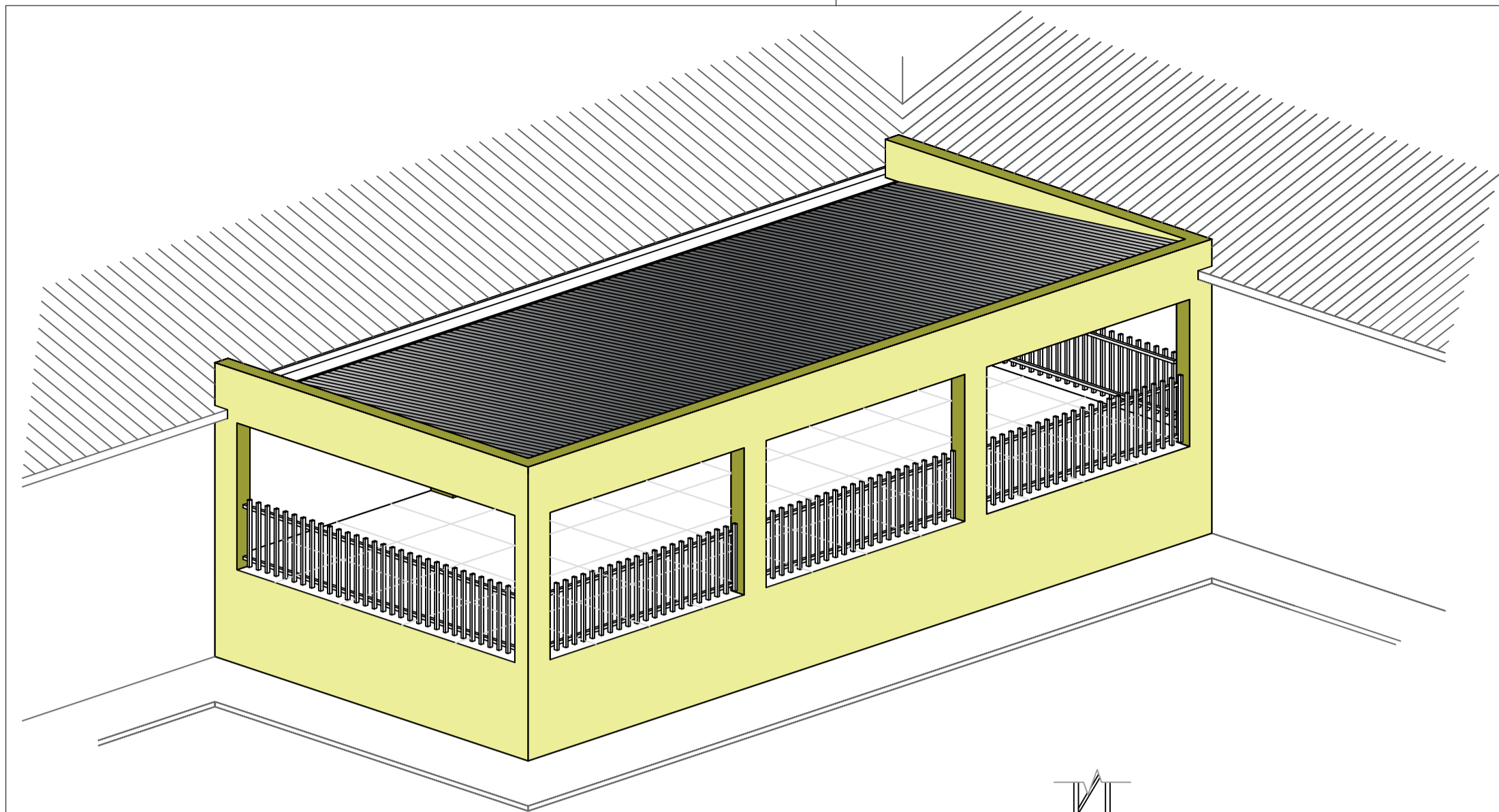
PERSPECTIVA VARANDA MATERNAL ESCALA - 1/75
