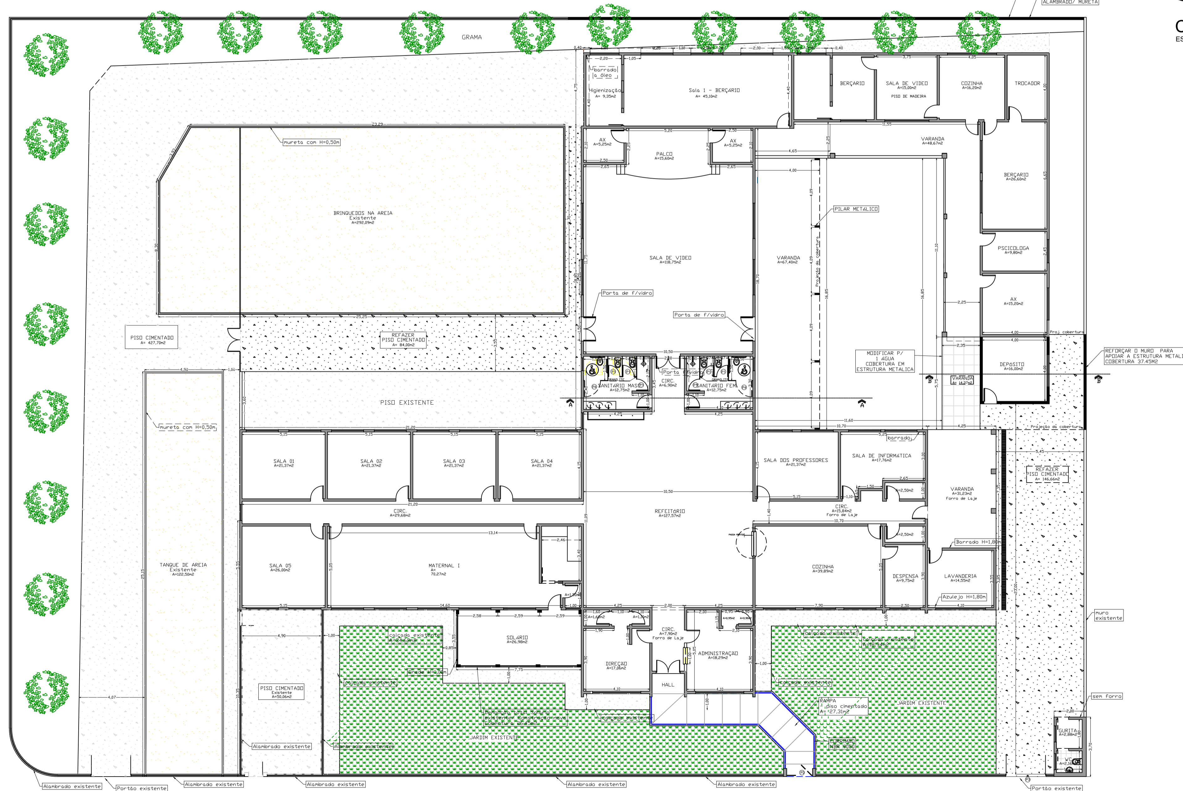
Planta Baixa ESCALA - 1/150
