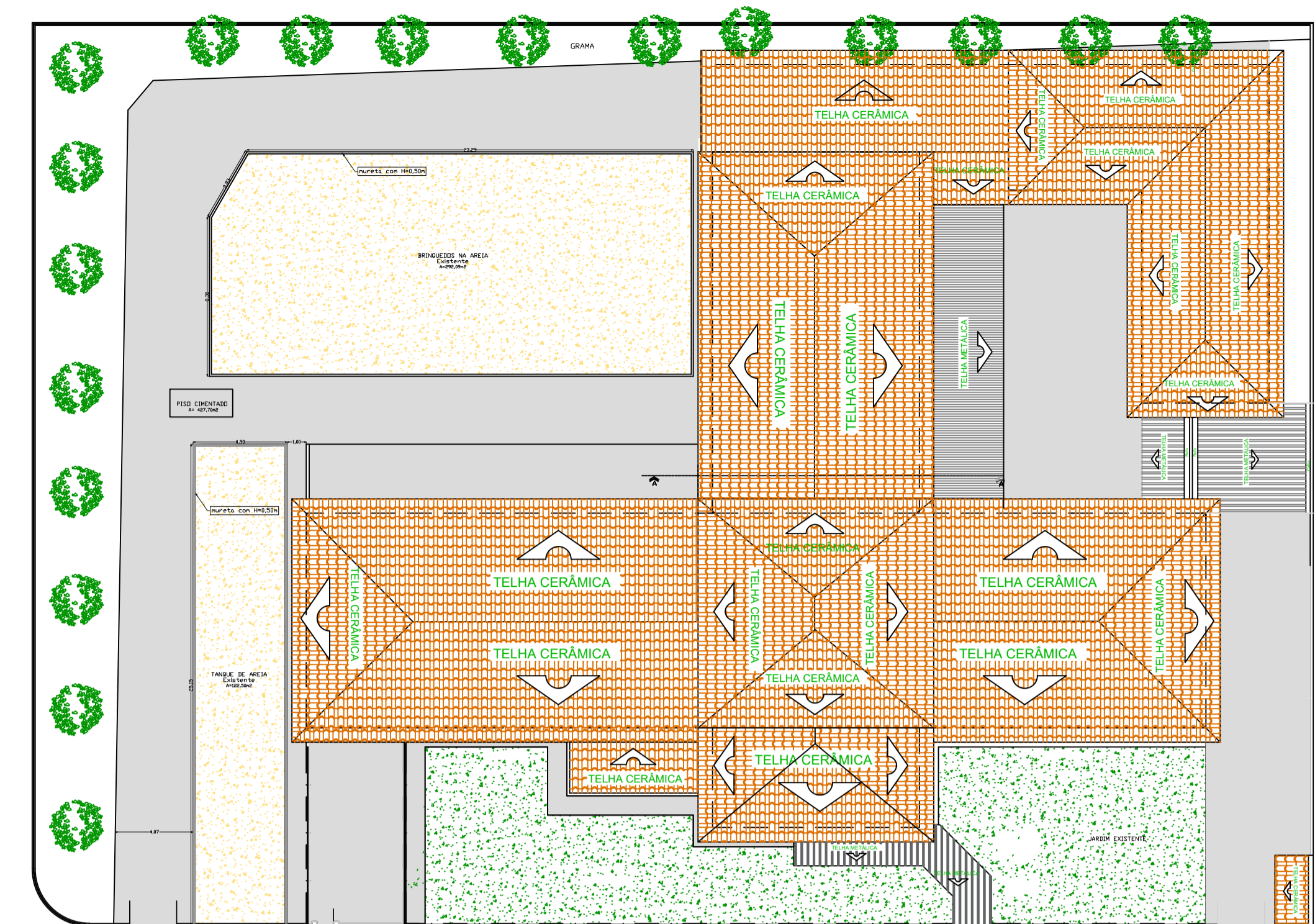
COBERTURA E IMPLANTAÇÃO ESCALA - 1/250
