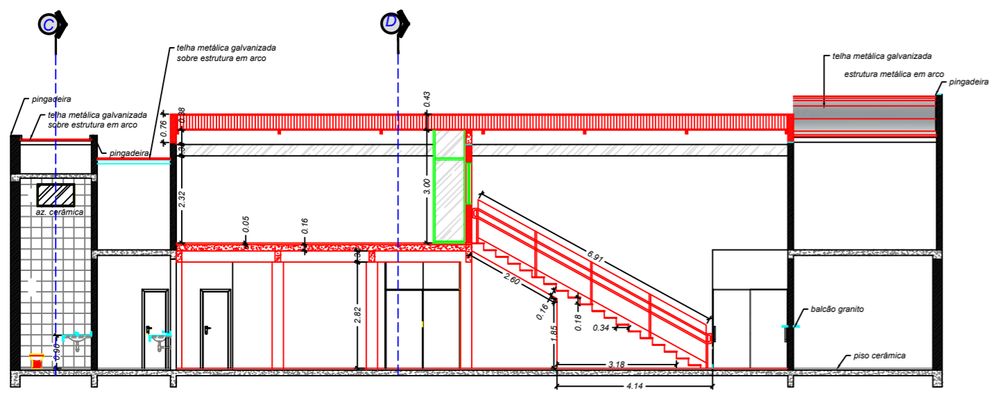
Corte bb ESCALA 1:75
