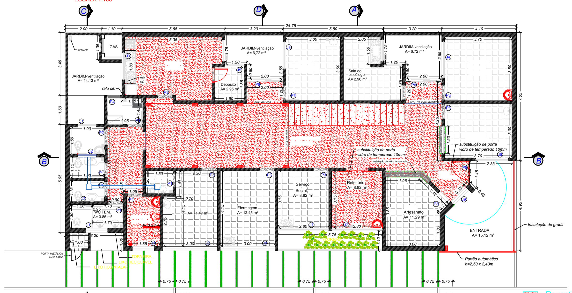
PLANTA - Piso Térrio - 242,44m 2 ESCALA 1:100
