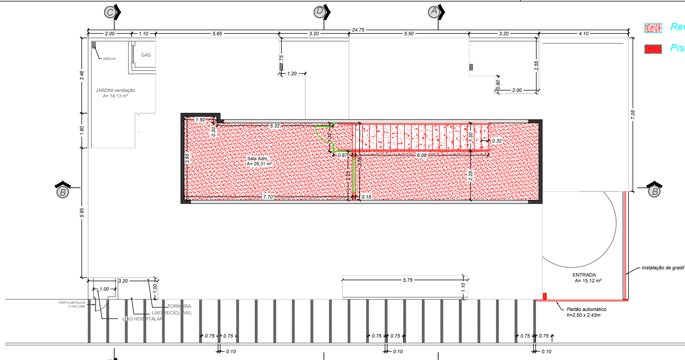
PLANTA - Piso Superior - 28,31m 2 ESCALA 1:100
