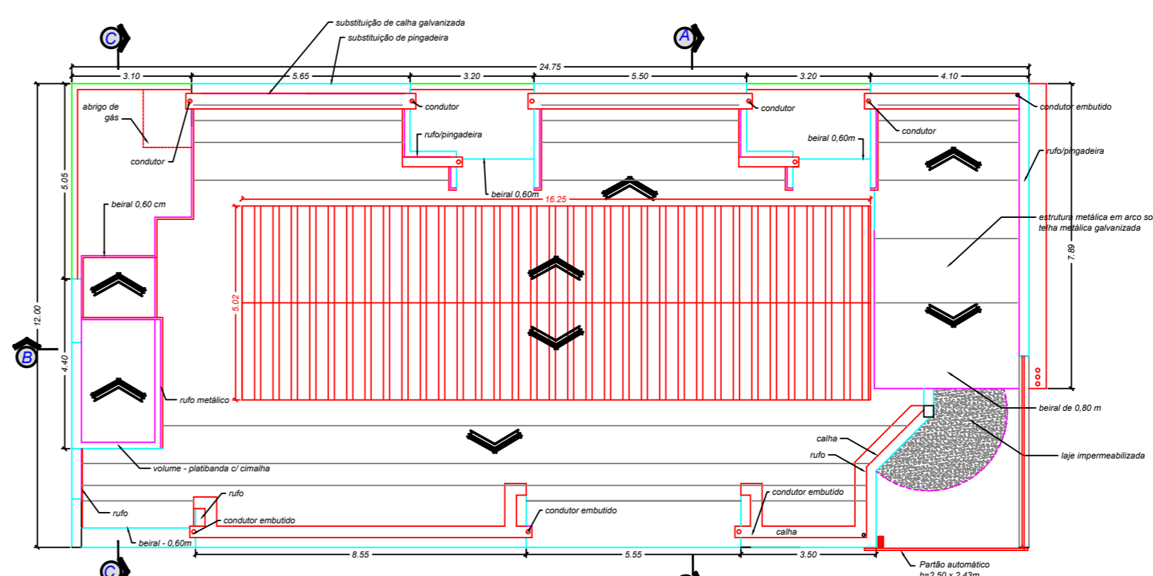
Cobertura ESCALA 1:100
