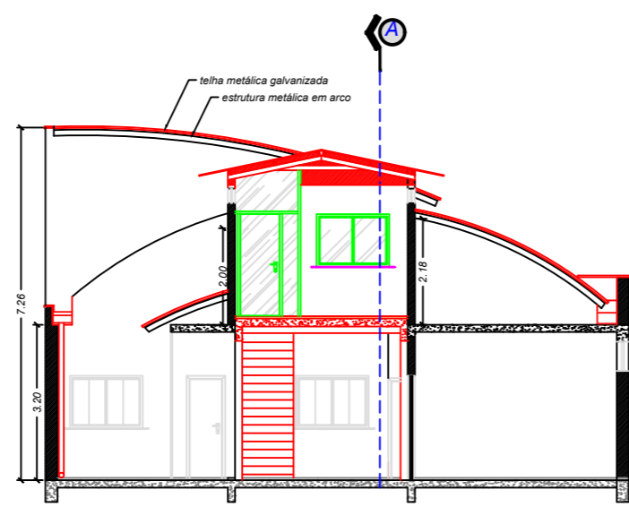
Corte dd ESCALA 1:75
