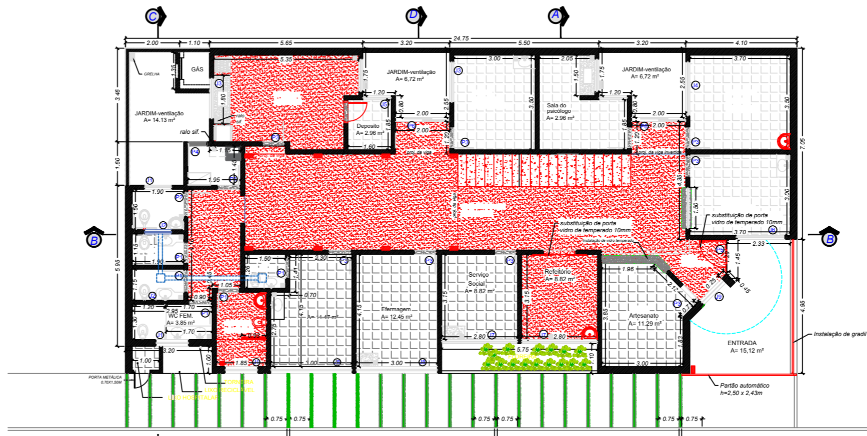
PLANTA - Piso Térrio - 242,44m2 ESCALA 1:75
