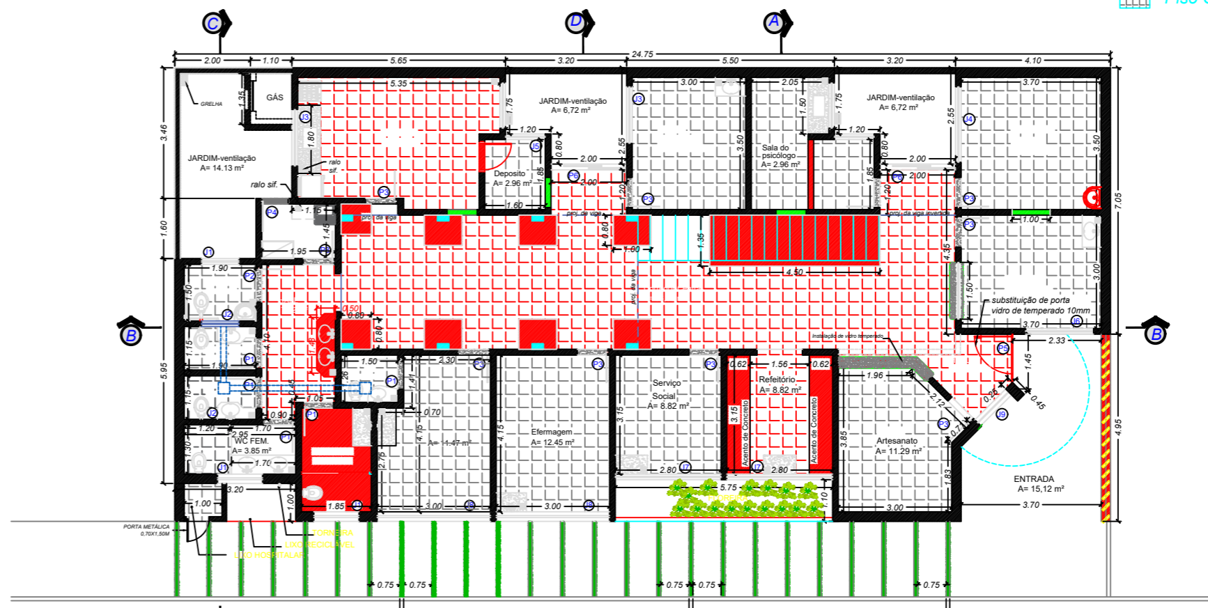
PLANTA - 242,44m2 ESCALA 1:75
