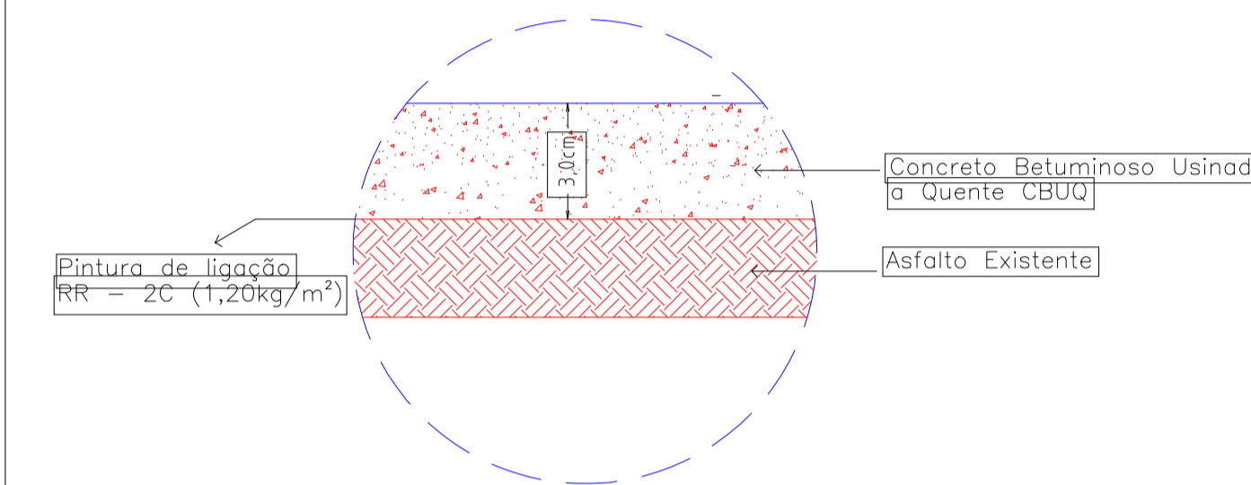
Detalhe CBUQ - Concreto Betuminoso usinado a quente
