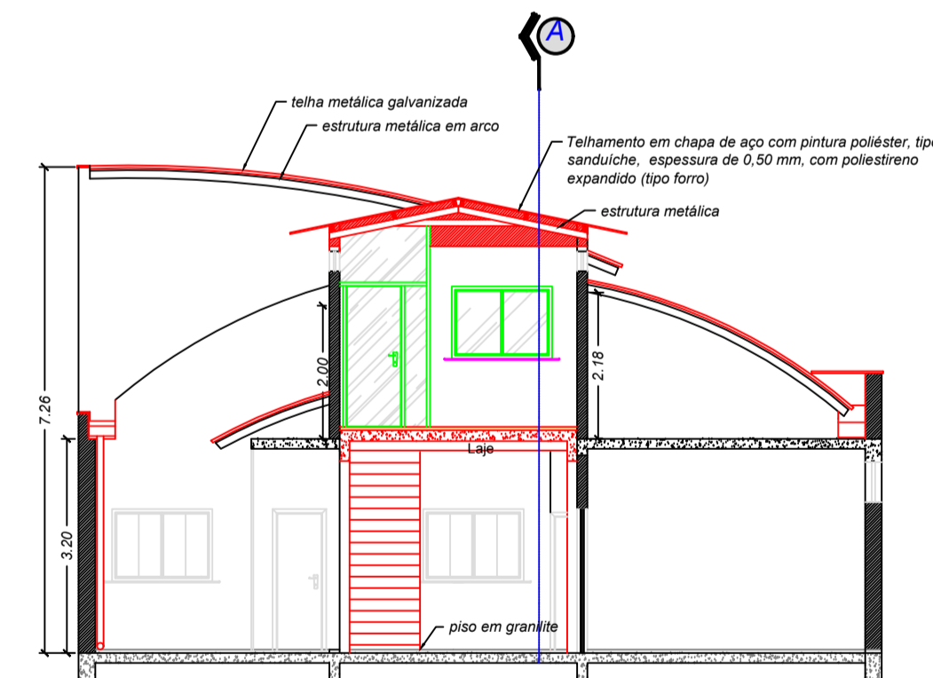
Corte dd ESCALA 1:100
