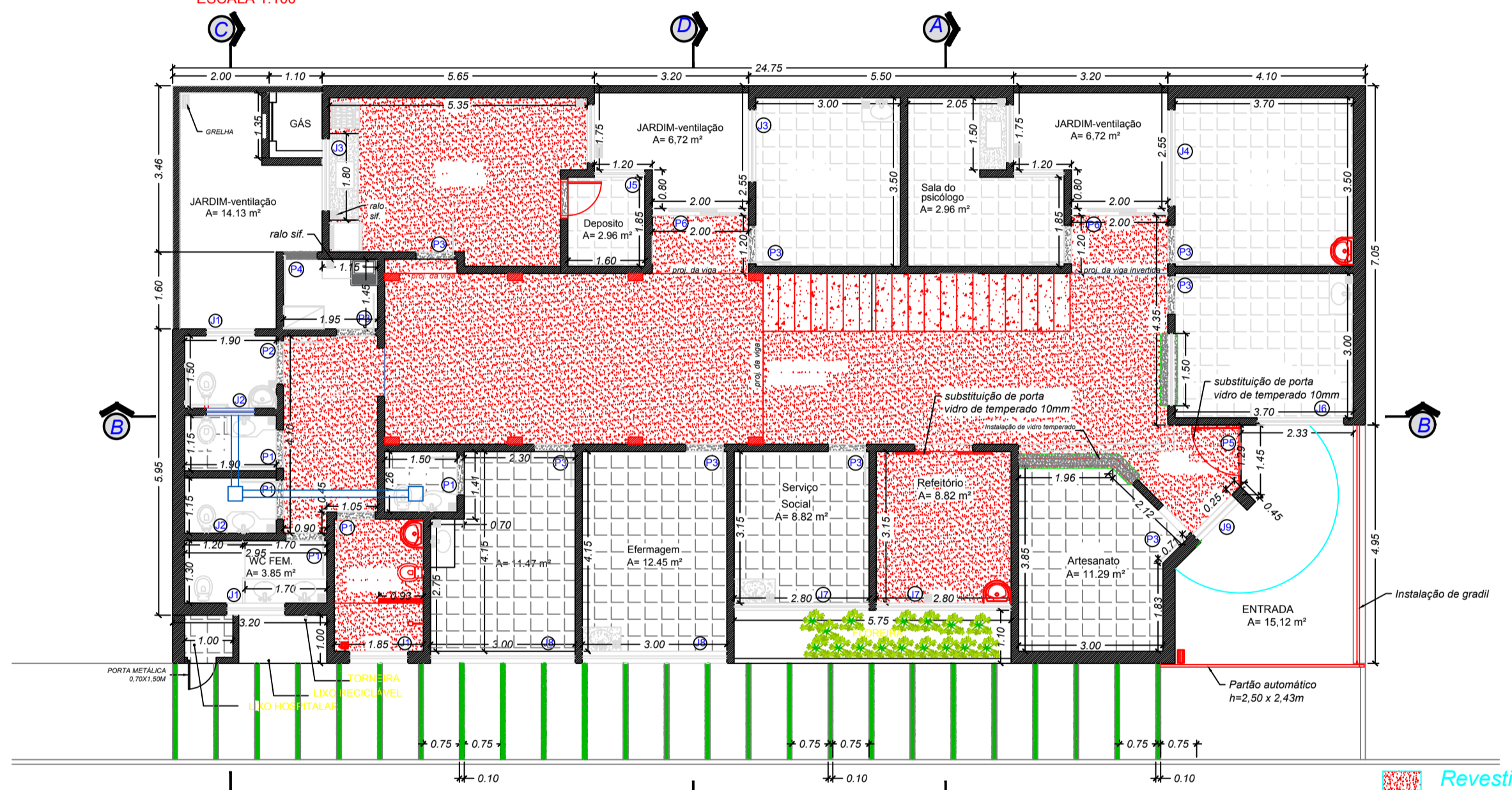
PLANTA - Piso Térrio - 242,44m 2 ESCALA 1:100
