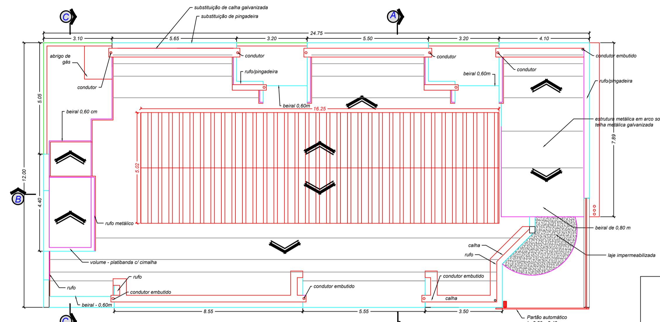
Cobertura ESCALA 1:100
