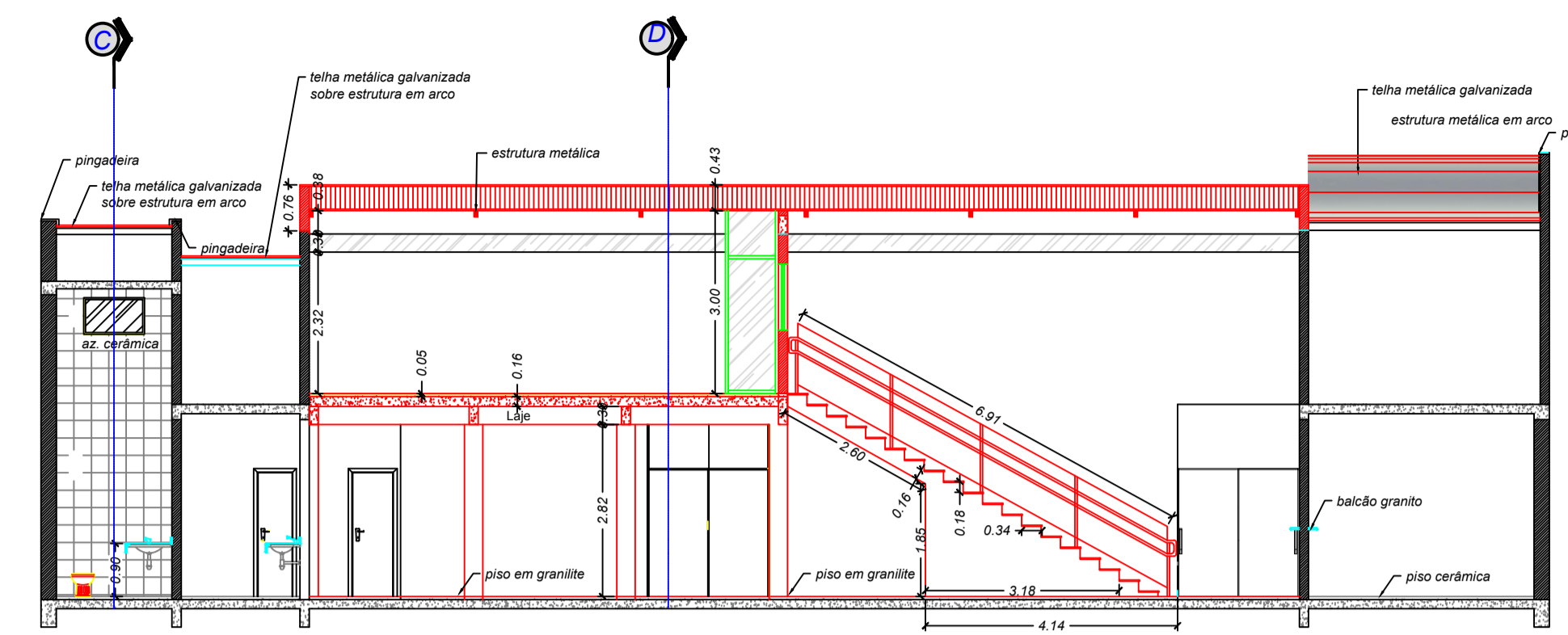
Corte bb ESCALA 1:00
